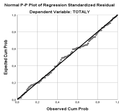
GAMBAR 3.1 Grafik P-Plot
