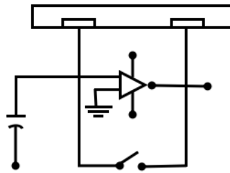
Gambar 2.7 Rangkaian Sensor Kapasitif [23]
