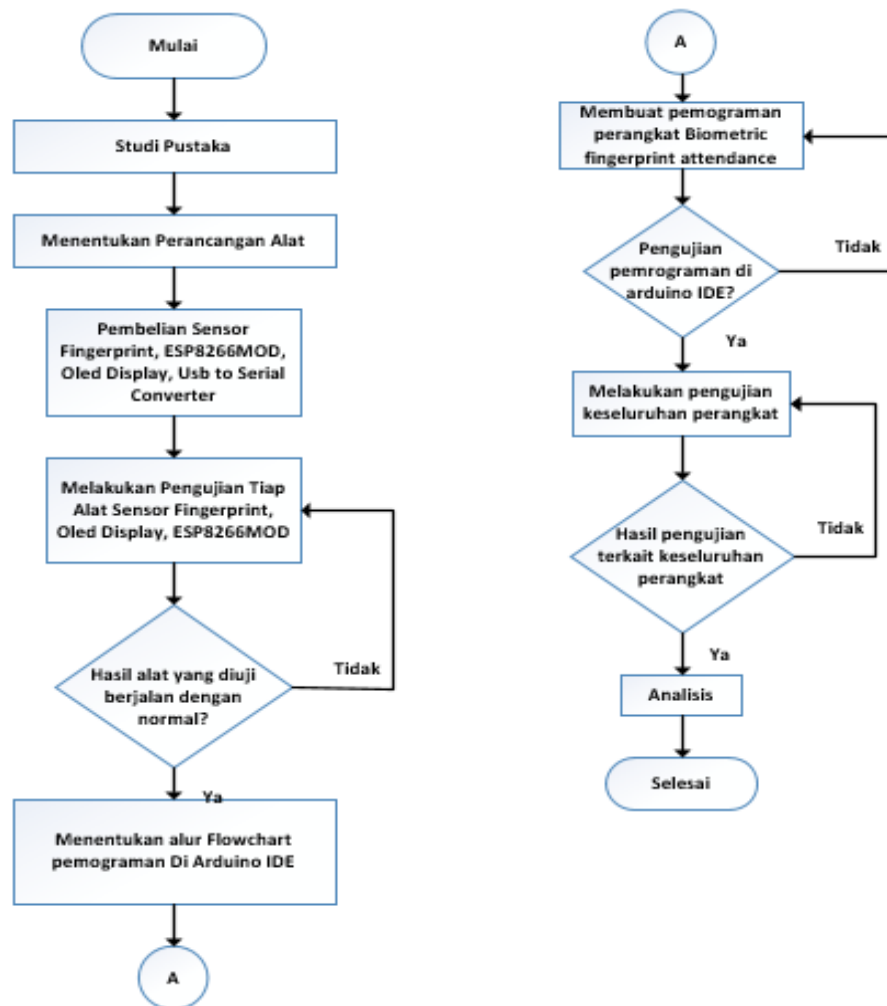
Gambar 3.1 Flowchart Pengerjaan Proyek Akhir.
