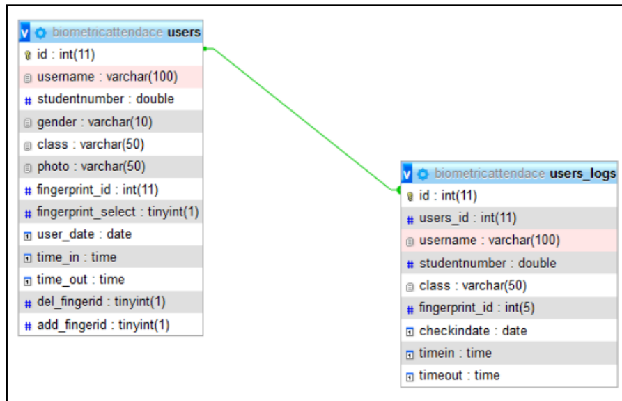
Gambar 3.13 Tabel Relasi Database
