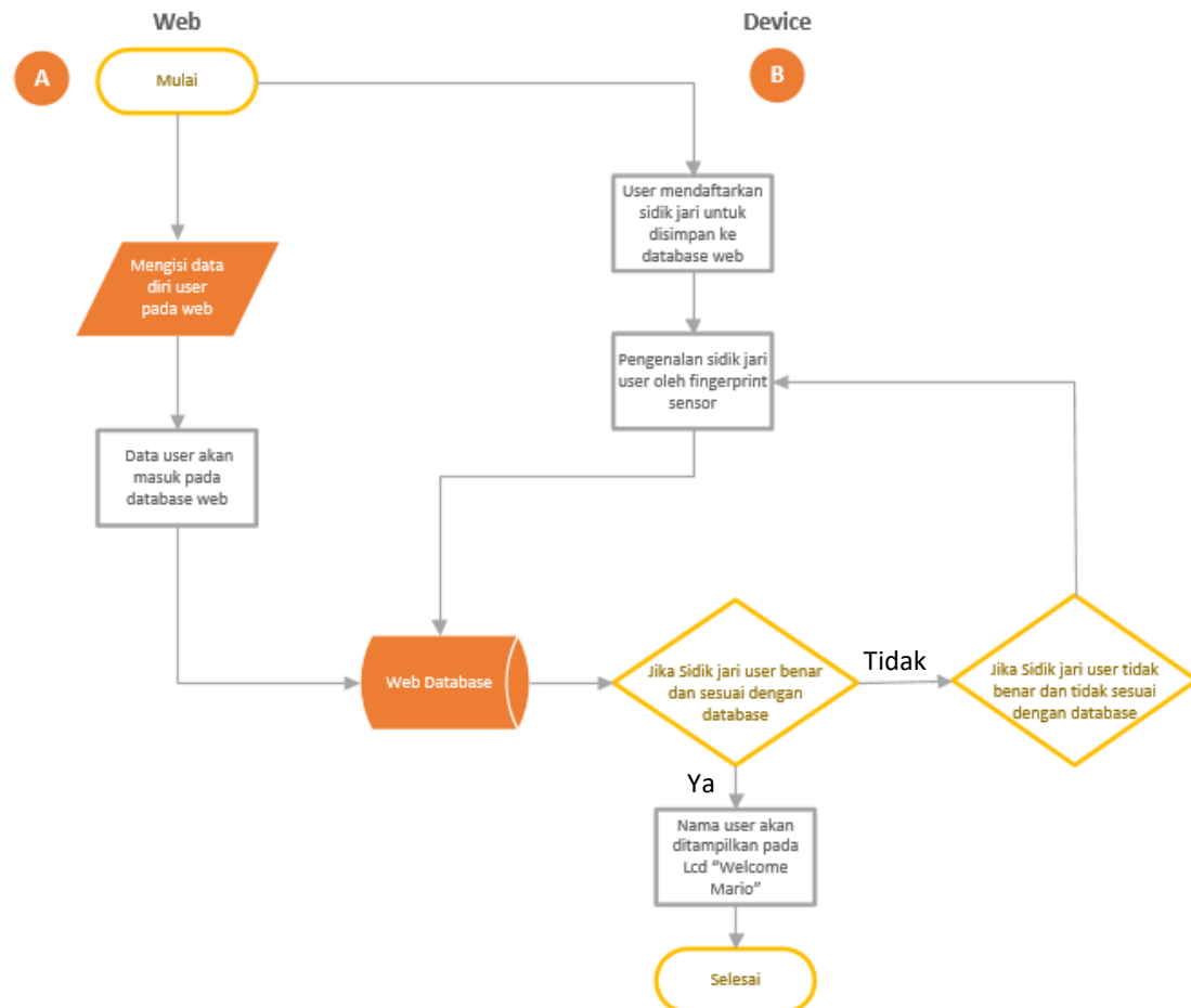
Gambar 3.3 Flowchart Kerja Keseluruhan Sistem.
