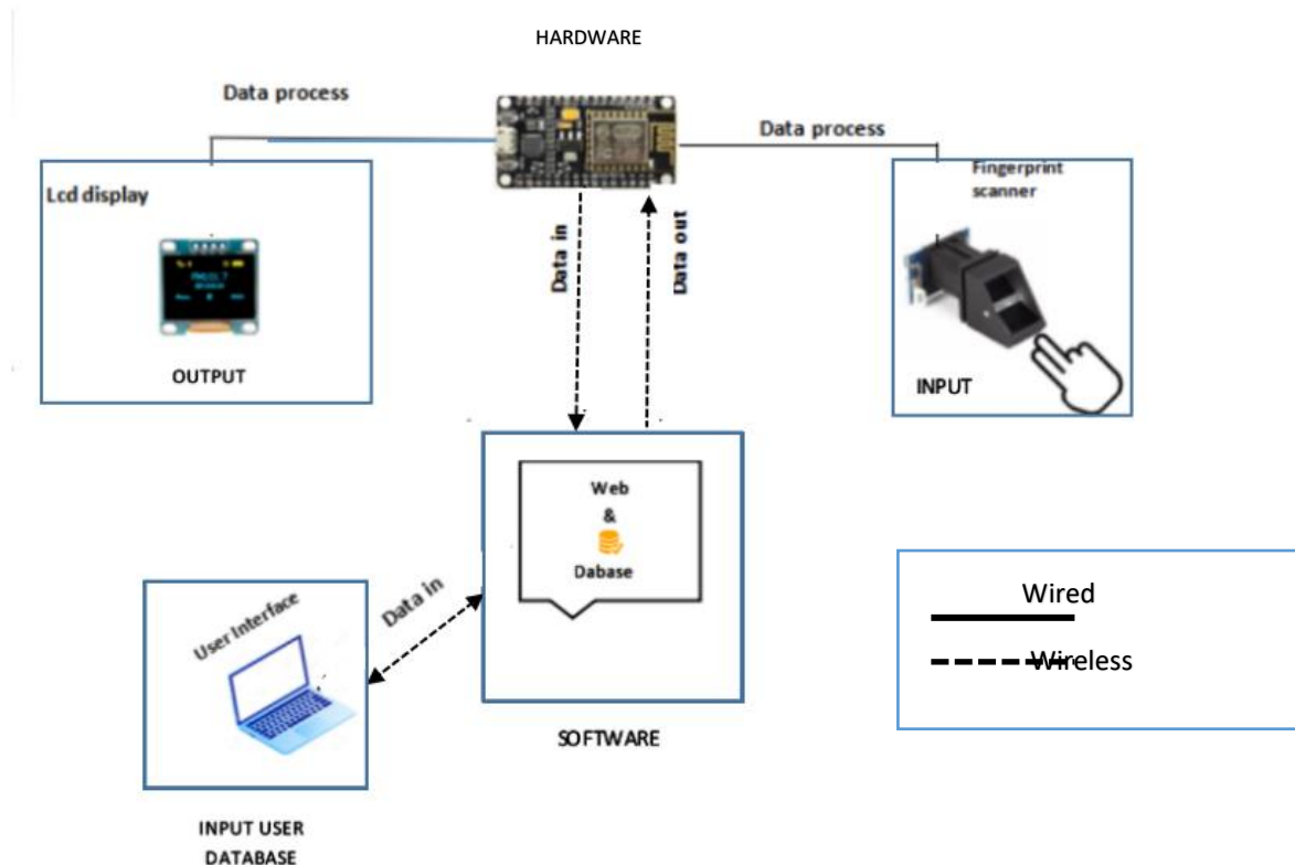
Gambar 3.2 Blog Diagram Keseluruhan Sistem Biometric Fingerprint Attendance Dan Web Monitoring Sistem.
