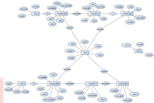
Gambar 3- 13 ER-D
