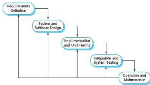
Gambar 1- 1 Metode Pengerjaan
