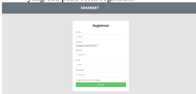
Gambar 4- 2 Tampilan Registrasi
