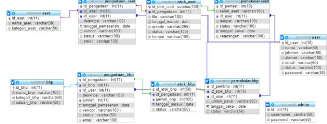
Gambar 3- 14 Skema Relasi
