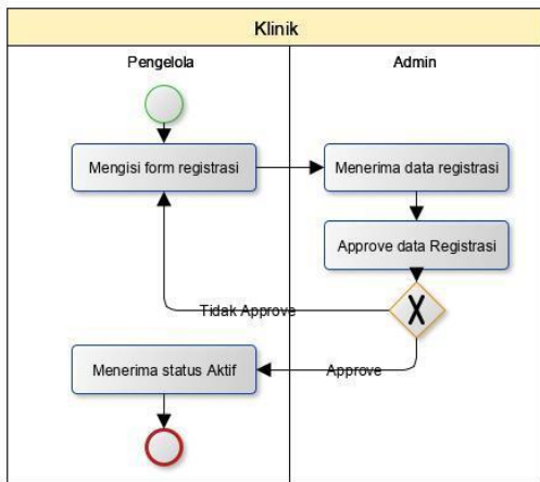
Gambar 3- 5 Registrasi Petugas
