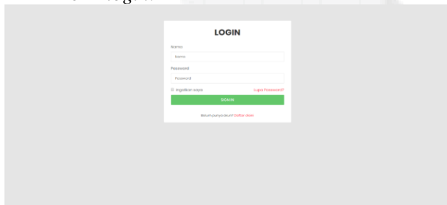
Gambar 4- 3 Tampilan Login
