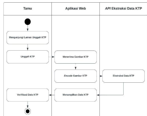
Gambar 3. 1 activity diagram fitur ekstraksi data citra KTP
