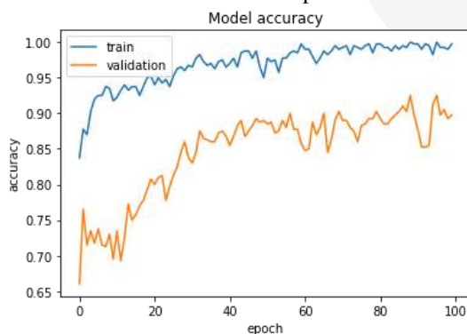
Gambar 3. 3 Grafik pertumbuhan akurasi selama proses latih
