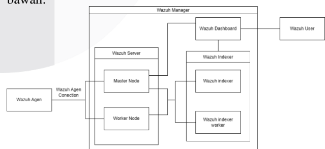
GAMBAR 3 Infrastruktur Wazuh
