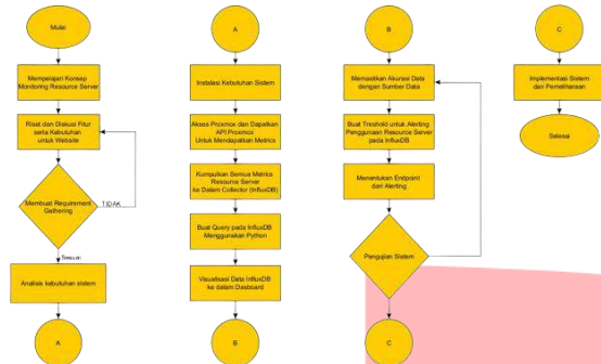
GAMBAR 2. 1 Flowchart Perancangan Sistem
