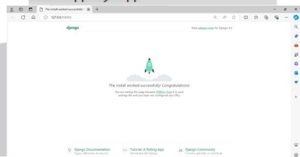
GAMBAR 2. 2 Django
