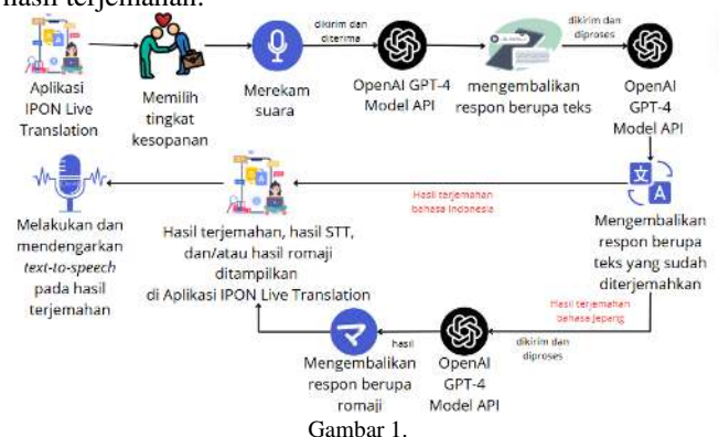
Gambar 1. Arsitektur IPON Live Translation
