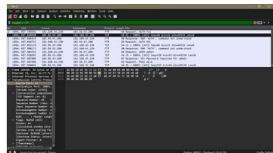
GAMBAR 4.6 Hasil FTP Tanpa VPN
