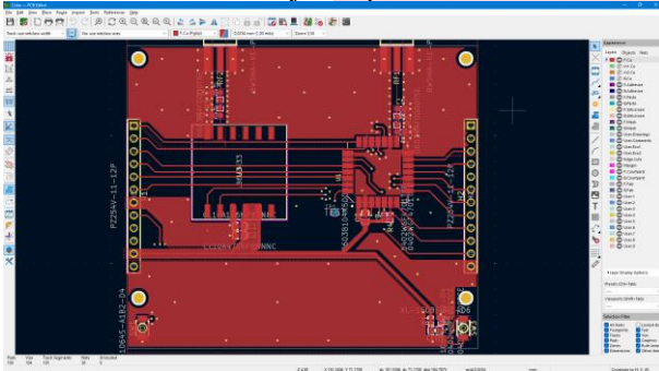
GAMBAR 15 Lapisan 1
