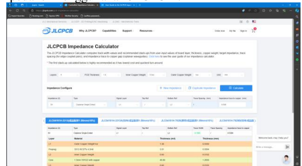
GAMBAR 13 Kalkulator Impedansi
