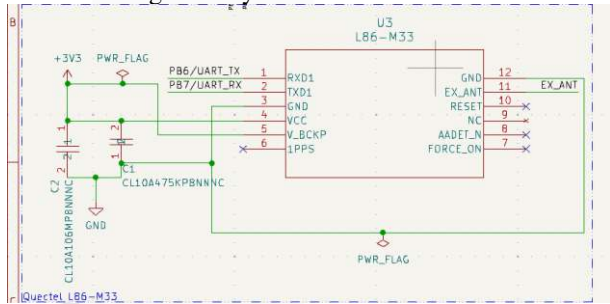
GAMBAR 8 Rangkaian Modul GPS
