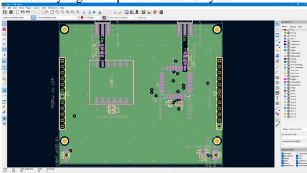
GAMBAR 16 Lapisan 2
