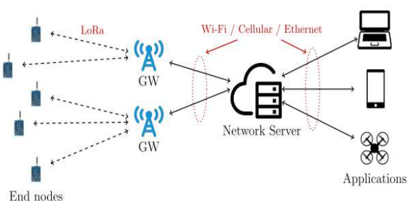
GAMBAR 1 Arsitektur LoRaWAN
