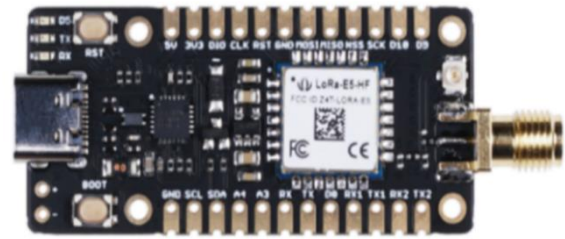
GAMBAR 2 LoRa-E5 Mini
