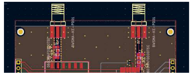
GAMBAR 12 Jalur Antena
