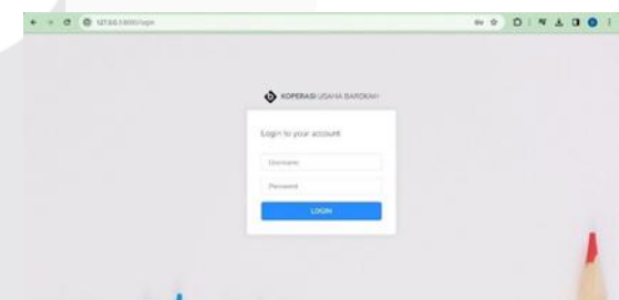
GAMBAR 8 Halaman Login
