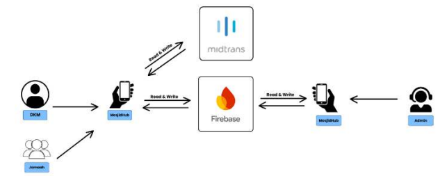
GAMBAR 1 ARSITEKTUR APLIKASI
