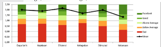
Gambar 27 Grafik Benchmark
