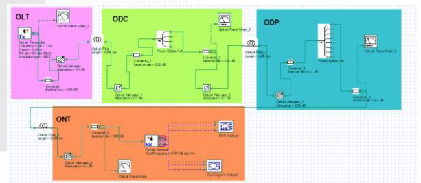
GAMBAR 4 SIMULASI ONT TERJAUH (DOWNSTREAM)
