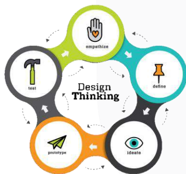
GAMBAR 1 Metode Pengerjaan
