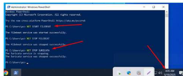
GAMBAR 4 Pengujian
