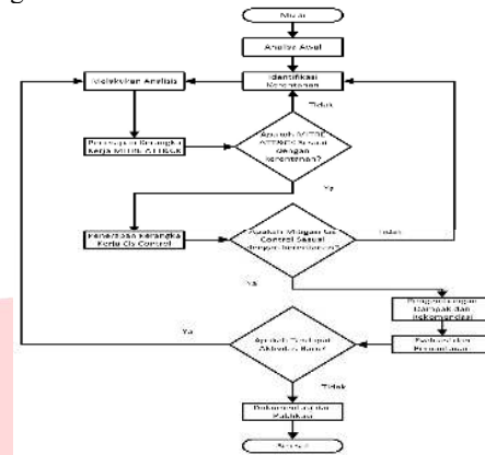
GAMBAR 1 Alur Kerja
