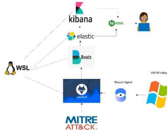
GAMBAR 3 Gambaran Sistem
