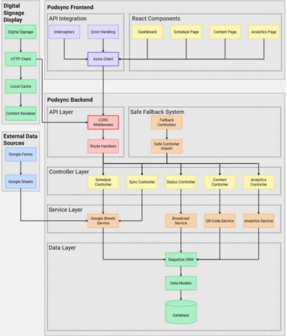
GAMBAR 11 Diagram Arsitektur API
