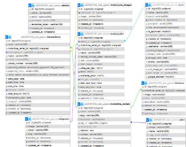
GAMBAR 3 ERD Webgassor
