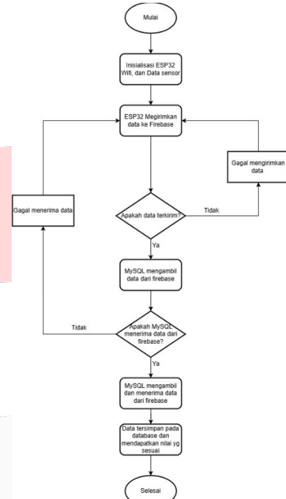
GAMBAR 3 Diagram Alir Pengiriman Data
