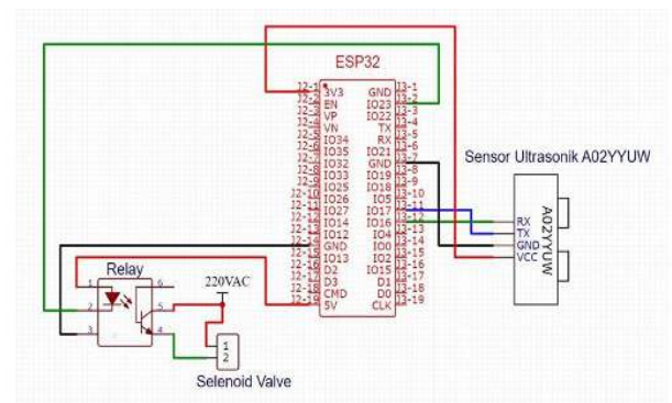
GAMBAR 2 Simulasi sistem
