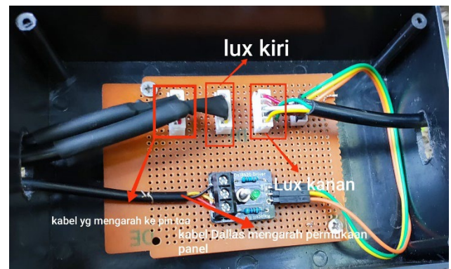
GAMBAR 4 Casing kotak sensor Cahaya dan suhu
