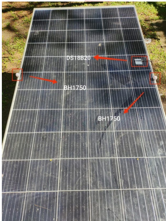
GAMBAR 3 sensor Cahaya (BH1750) dan suhu (DS18B20)
