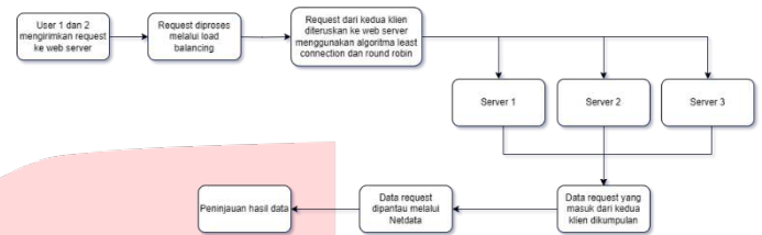
GAMBAR 1 Alur Kerja Sistem Load Balancing
