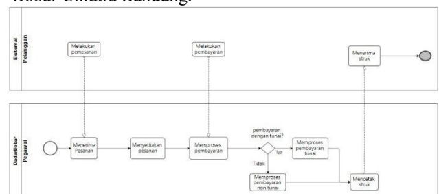
GAMBAR 3 BPMN
