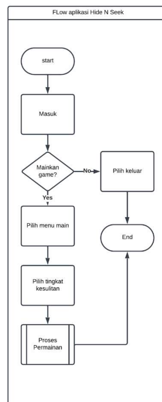
GAMBAR 2 Alur Umum Game
