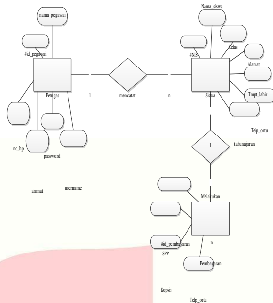
Gambar 3-7 ERD
