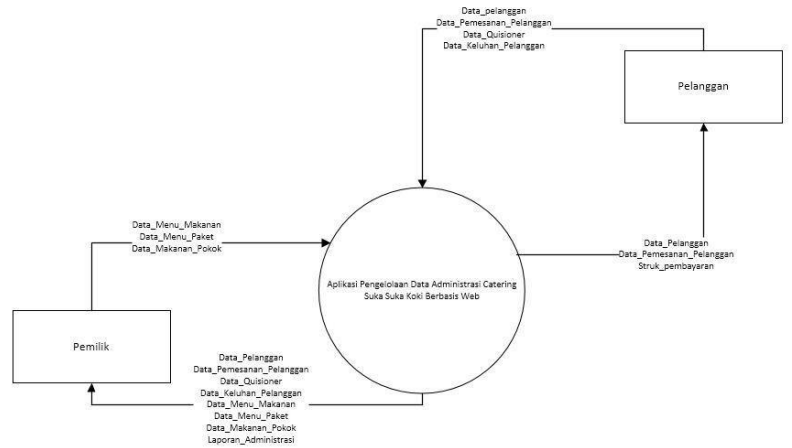
Gambar 3 Diagram Konteks
