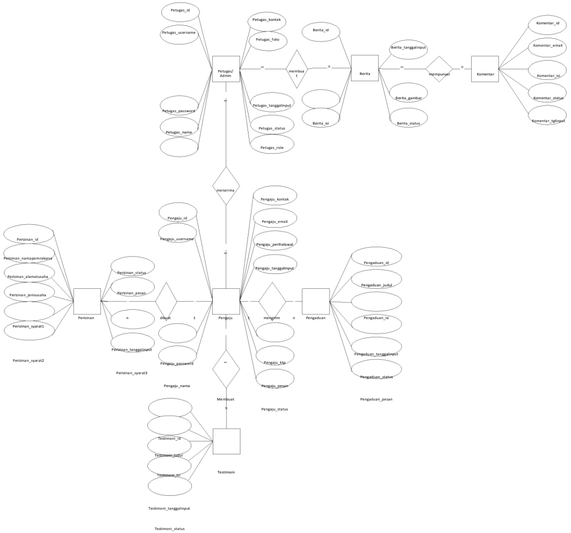
Gambar 3.6 ERD
