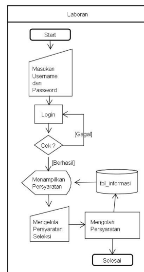
Gambar 5 Flowmap Usulan Mengelola Informasi Seleksi
