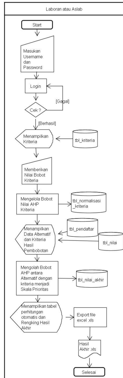
Gambar 9 Flowmap Usulan Perhitungan AHP untuk Hasil Akhir
