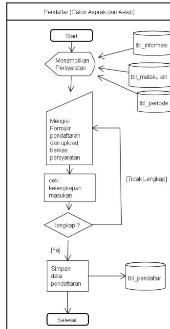
Gambar 7 Flowmap Usulan Pendaftaran Asisten
