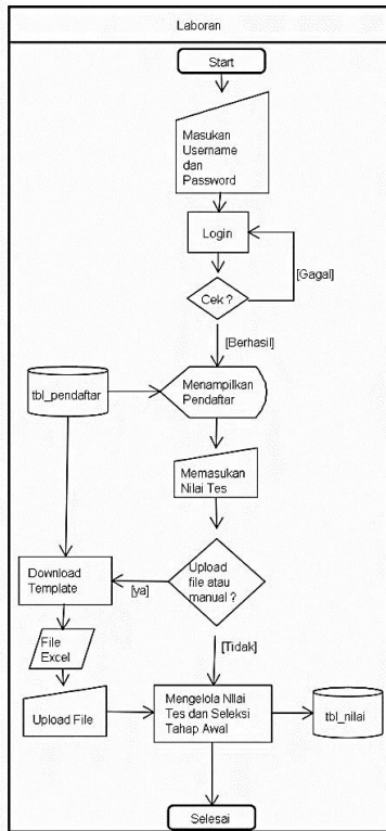
Gambar 8 Flowmap Usulan Kelola Nilai Alternatif
