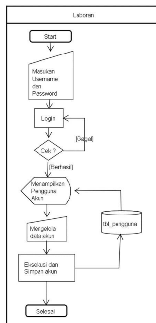
Gambar 2 Flowmap Usulan Pengelolaan Admin
