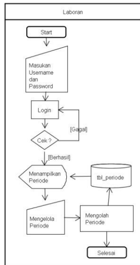
Gambar 3 Flowmap Usulan Kelola Periode
