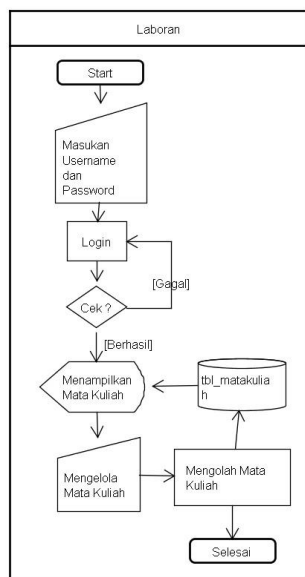
Gambar 4 Flowmap Usulan Kelola Mata Kuliah
