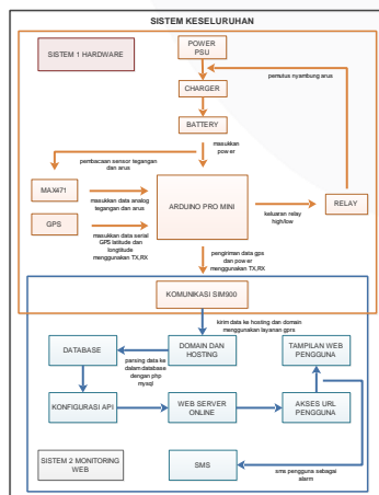
Gambar 3-1 Blok Diagram Sistem Usulan Keseluruhan
