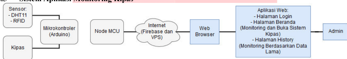
Gambar 2 Perancangan Sistem Aplikasi Monitoring Kipas
