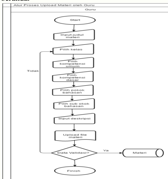
Gambar 3. 6 Flowmap Usulan Input Data Materi Oleh Guru
