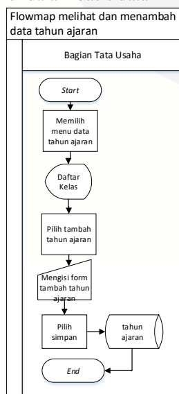
Gambar 3. 16 Flowmap menambah tahun ajaran
