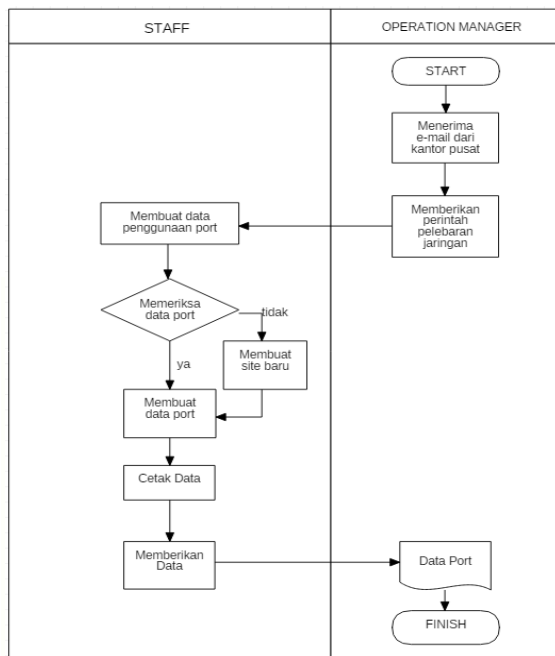
Gambar 3-1 Flowmap Proses Pelebaran Jaringan
