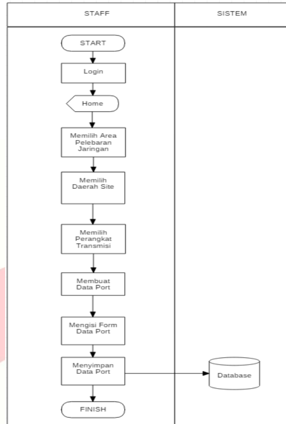
Gambar 3-4 Flowmap Pembuatan Data Port
