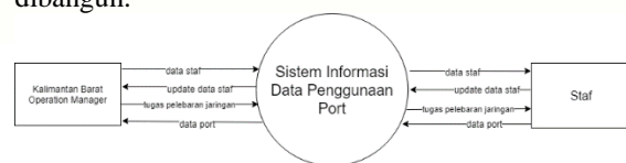
Gambar 3-5 Diagram konteks
