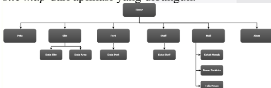
Gambar 3-8 Site Map Aplikasi
