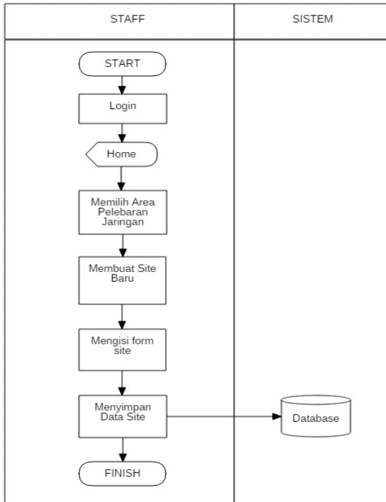
Gambar 3-3 Flowmap Proses Pembuatan Site Baru
