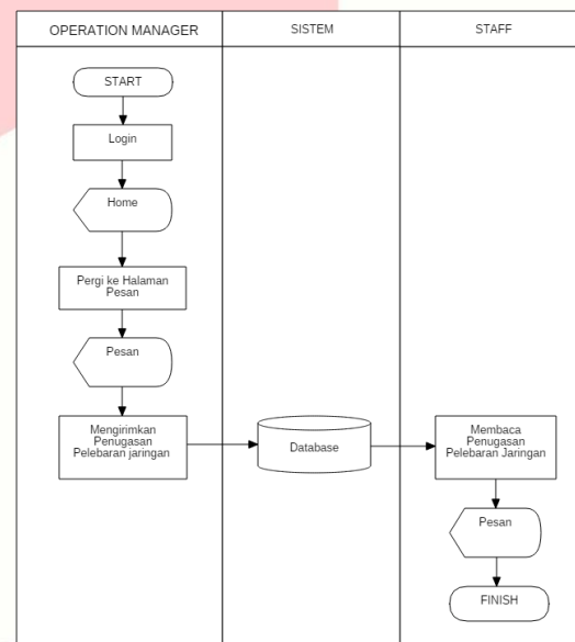
Gambar 3-2 Flowmap Proses Pelebaran Jaringan Baru Usulan
