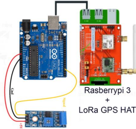
Gambar 4. 4 Skema Node Lora
