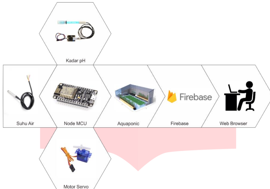
Gambar 3.1 Skema Sistem
