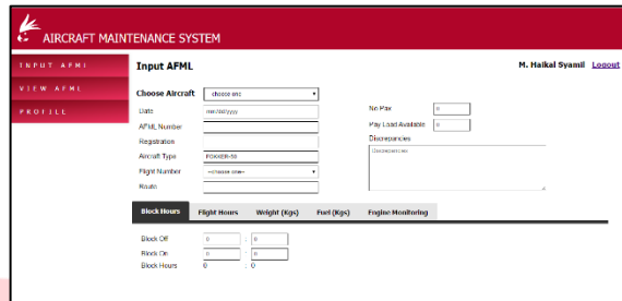
Gambar 4 Tampilan Input AFML
