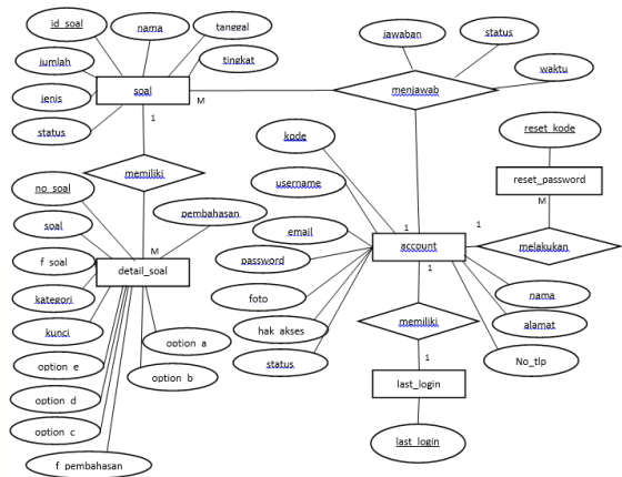
Gambar 3-6 Skema Relasi
