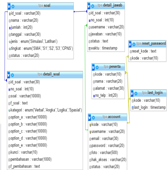
Gambar 3-7 Skema Relasi
