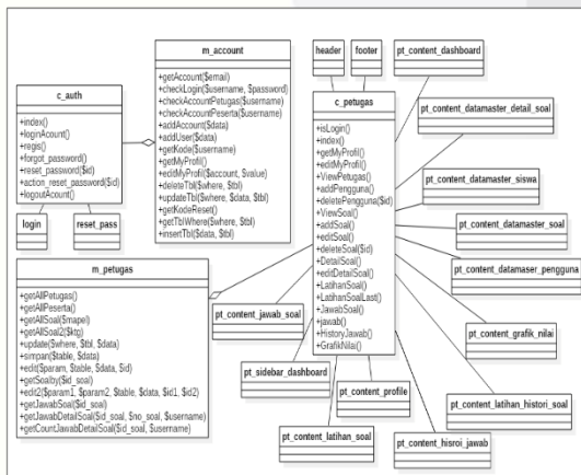
Gambar 3-5 Diagram Kelas
