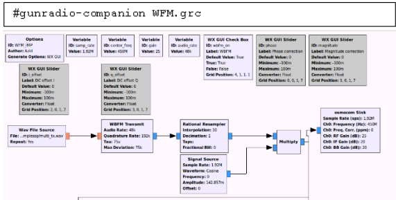
Gambar 4.5-1 WFM.grc
