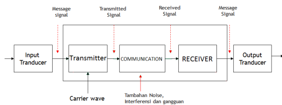
Gambar 2.1-1 Skema Dasar Komunikasi Radio
