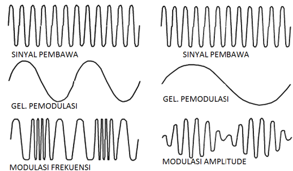
Gambar 2.1-3 Modulasi Amplitude dan Frekuensi
