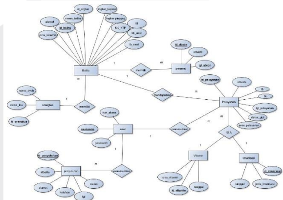
Gambar 5 ER Diagram
