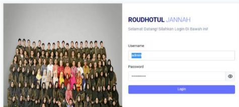
GAMBAR 1-6 Implementasi Login
