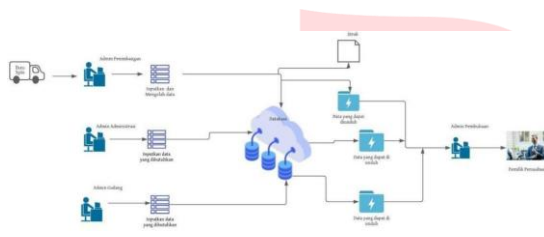
Gambar 3. 3 blok diagram sistem
