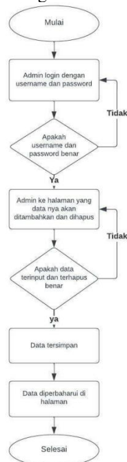
Gambar 3. 9 Alur Hapus dan Input Data
