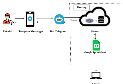
Gambar 2 Blok Diagram Sistem
