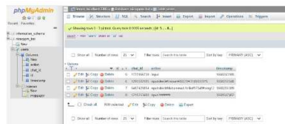
Gambar 6 Tabel Database
