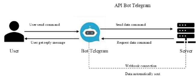
Gambar 1 Ilustrasi Webhook
