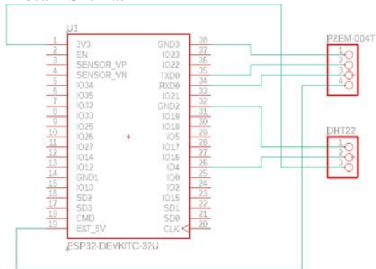
Gambar 4. Rangkaian Skematik Sistem
