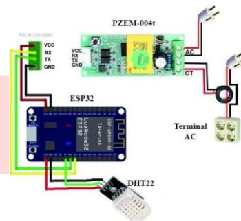
Gambar 2. Perancangan Sistem Kontroler Hardware
