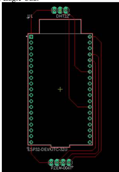
Gambar 3. Layout Pada PCB
