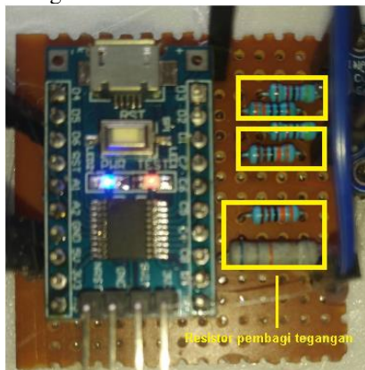
Gambar 3. 6 Rangkaian Sensor Tegangan
