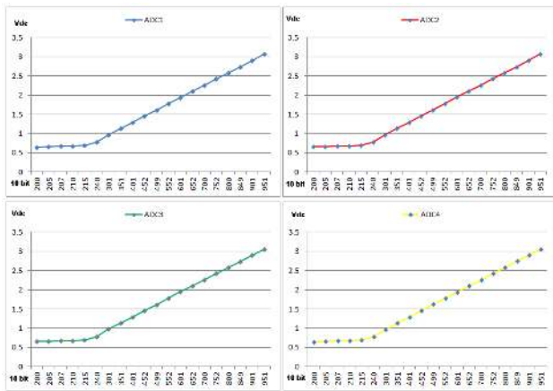
Gambar 3. 8 Grafik Pembacaan Tegangan Analog
