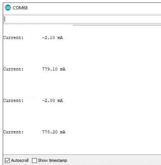
Gambar 3. 5 Pengujian Sensor Arus INA219
