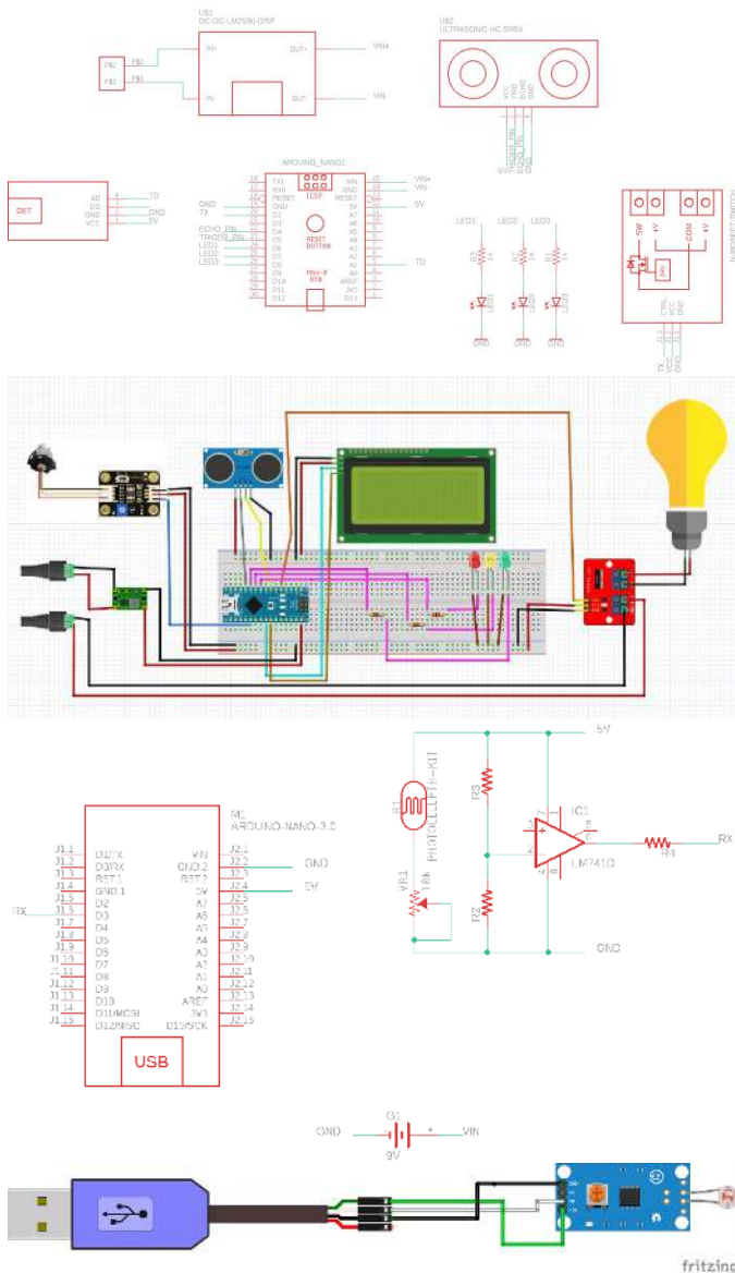
Gambar 9 Rangkaian Schematic
