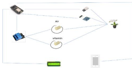
Gambar 3. 1 Perancangan keseluruhan
