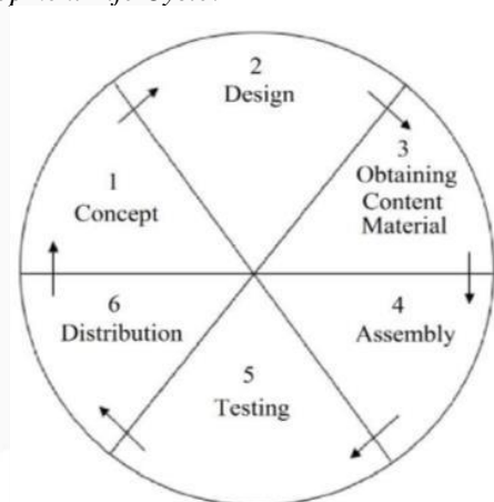
Gambar 2.3—1 Metode MDLC
