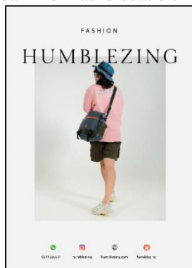
Gambar C—48 Informasi Humblezing
