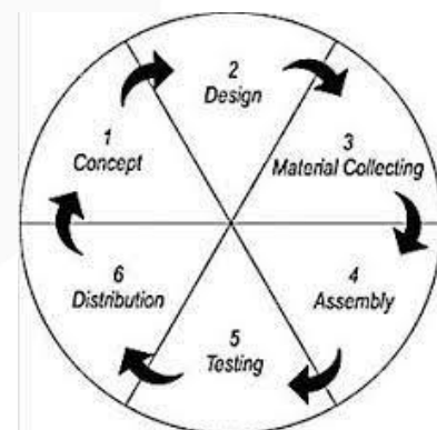
Gambar 1 Metodologi MDLC
