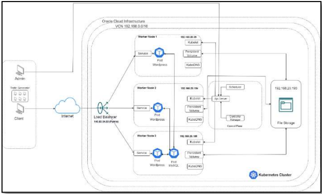
GAMBAR 3.2 Desain Sistem Perancangan
