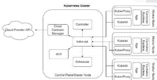
GAMBAR 2.1 Arsitektur Kubernetes
