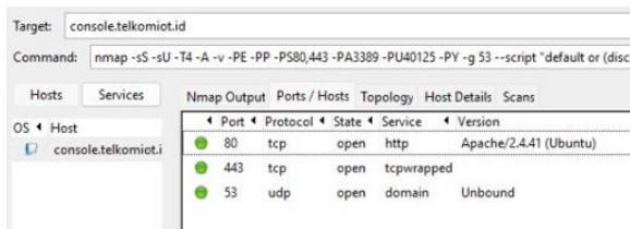
GAMBAR 4.1 Hasil Pengujian Nmap
