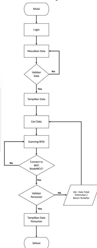
Gambar 3 Flowchart Cara Kerja Sistem
